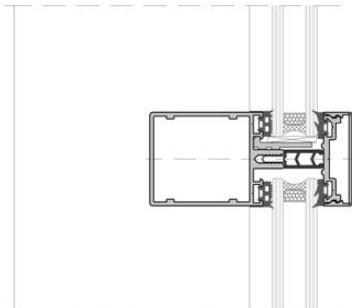
SECCION VERTICAL
