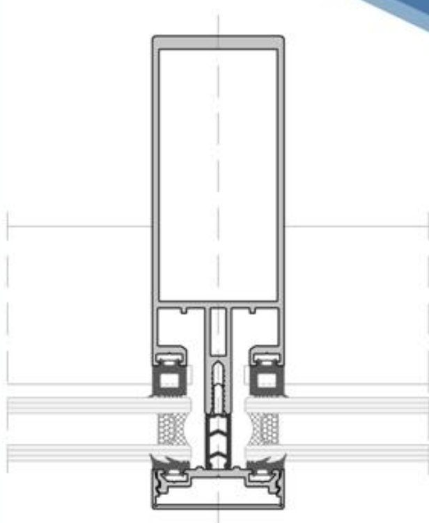
SECCION HORIZONTAL
