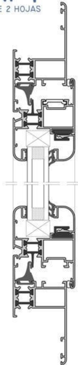
SECCION VERTICAL
