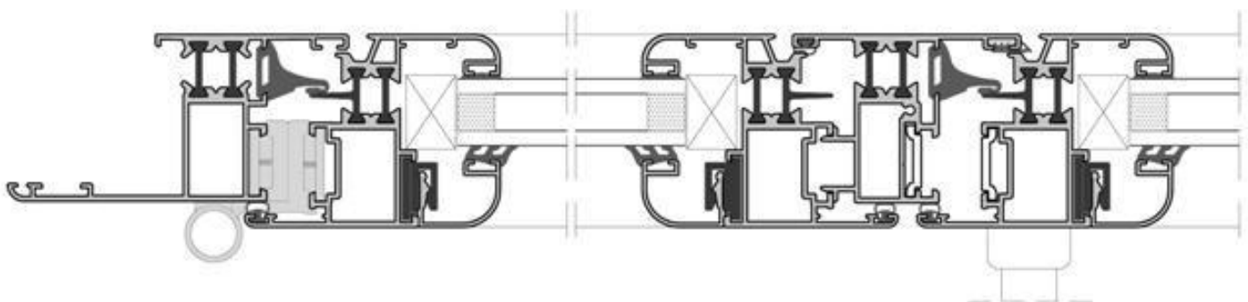
SECCION HORIZONTAL
